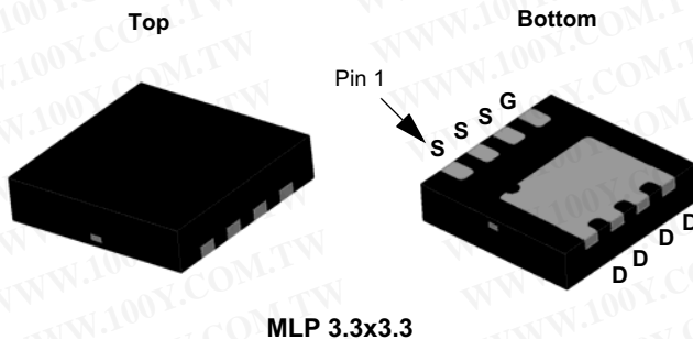
MLP 3.3x3.3
