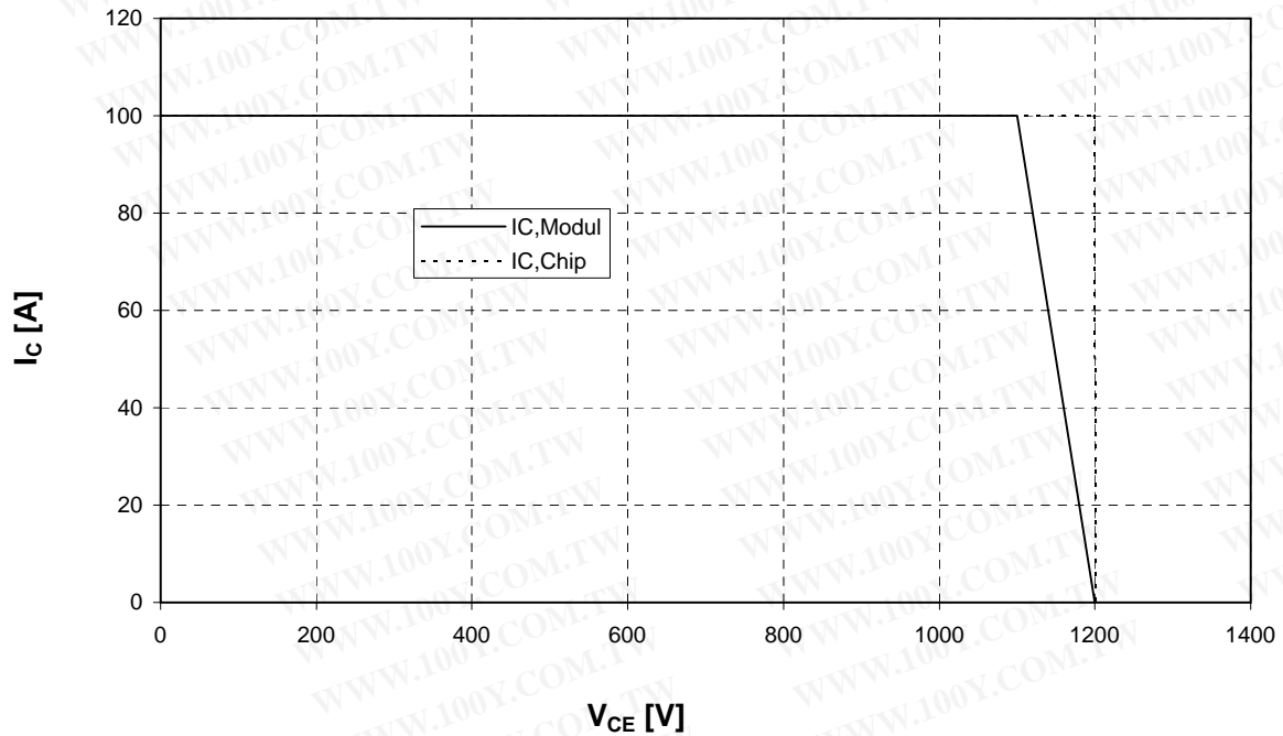
Sicherer Arbeitsbereich Wechsler. (RBSOA) \xi = f(V_{CE}) Reverse bias safe operating area Inverter (RBSOA) T_{vj} = 125^\circ\text{C} , V_{GE} = \pm 15\text{V} , R_G = 15 \text{ Ohm}
