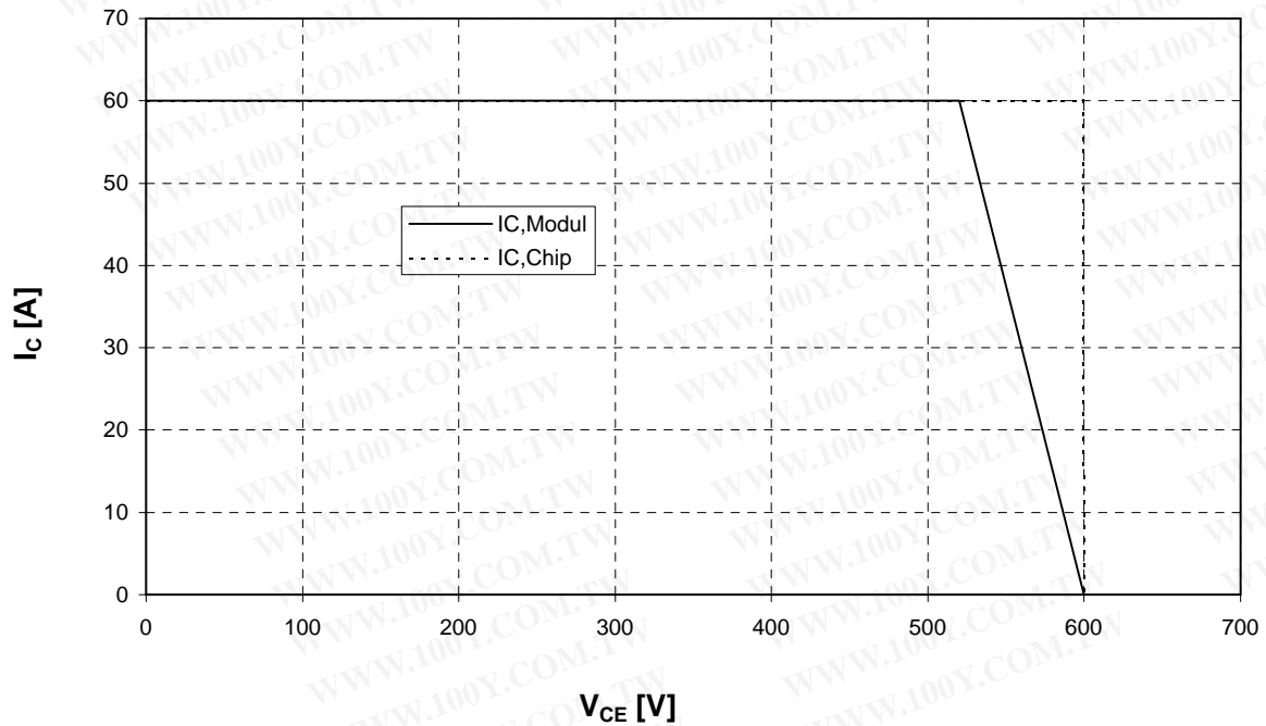
Sicherer Arbeitsbereich Wechsler. (RBSOA) I_c = f(V_{CE}) Reverse bias safe operating area Inverter (RBSOA) T_{vj} = 125^\circ\text{C} , V_{GE} = \pm 15\text{V} , R_G = 33 \text{ Ohm}
