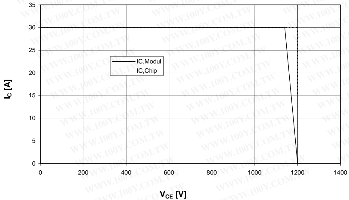
Sicherer Arbeitsbereich Wechsler. (RBSOA) I_C = f(V_{CE}) Reverse bias safe operating area Inverter (RBSOA) T_{vj} = 125^\circ\text{C} , V_{GE} = \pm 15\text{V} , R_G = 47 \text{ Ohm}
