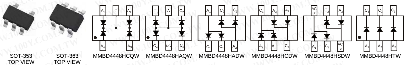
SOT353/SOT363
