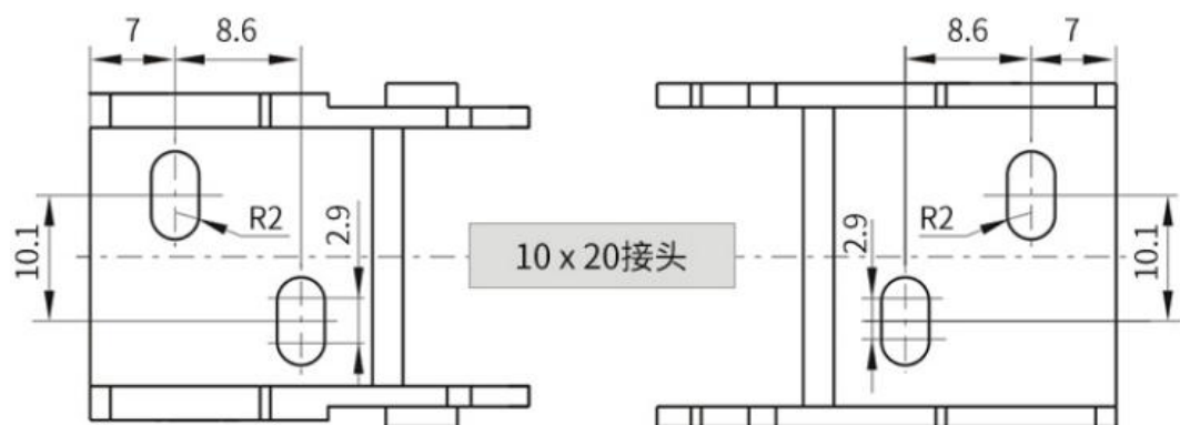
整体链接示意图
