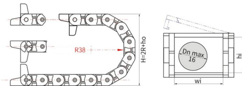
整体链接示意图
