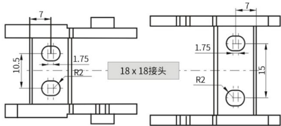
接头安装尺寸图
