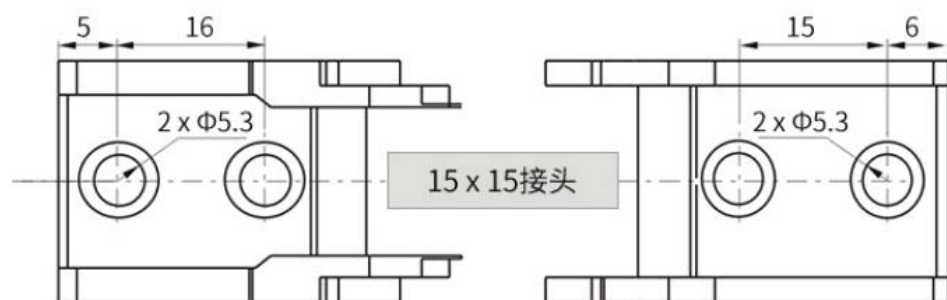
接头安装尺寸图
