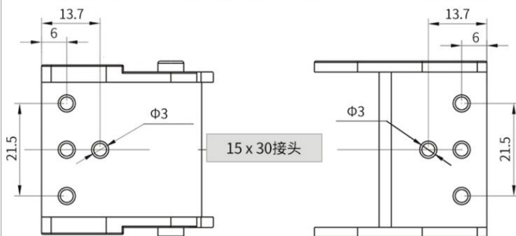
整体链接示意图
