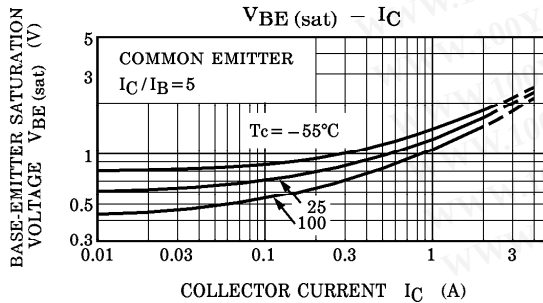
V_{BE(sat)} - I_C
