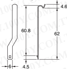
PFC-A1 (2 pieces per set)
