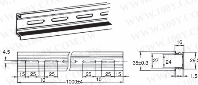
PFP-100N2 (Conforming to EN 50022)
