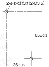
取り付け穴加工寸法 (TOP VIEW)
