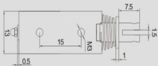
尺寸: 13*16.5*30mm
