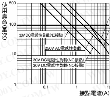
RJ1V 基準型
