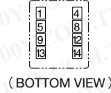
端子配置圖
