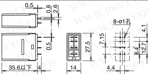
(圖片: RY2V-U 型)
