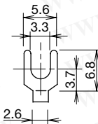
端子部形狀
