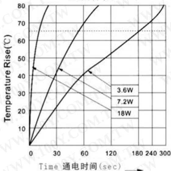
温度特性
