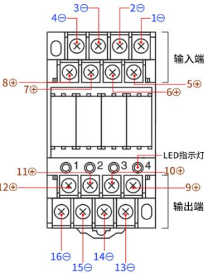
接线示意图
