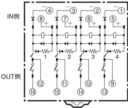
端子配置内部接线图
