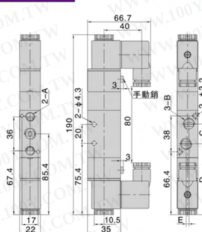
4V230DIN插座式
