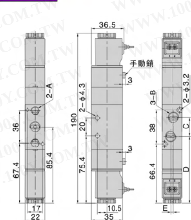
4V230出線式
