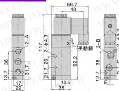
4V210DIN插座式
