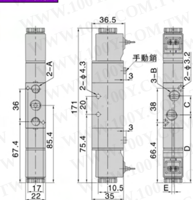
4V220出線式
