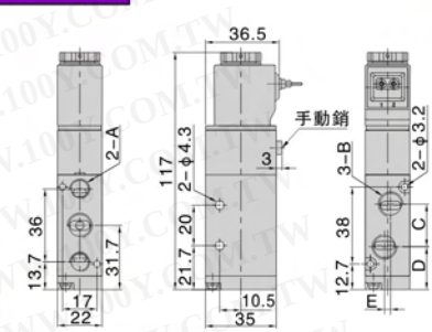
4V210出線式
