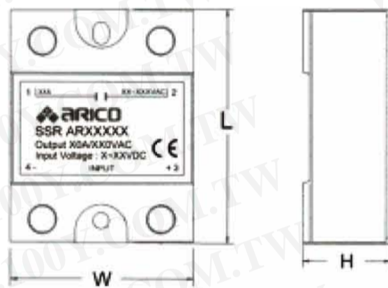
尺寸Dimension
