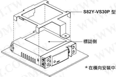
橫向安裝 (安裝配件*)
