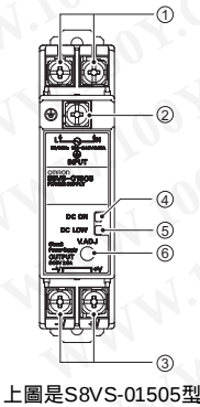
上圖是S8VS-01505型
