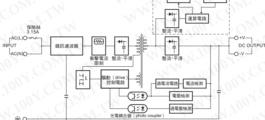
S8VS-06024 □ □ 型 ( 60W )
