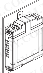
向上安裝 (安裝配件)
