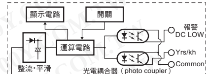
信號源型 ( S8VS-09024AP 型、S8VS-09024BP 型 )
