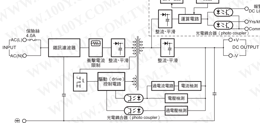
S8VS-09024 □ □ 型 ( 90W )
