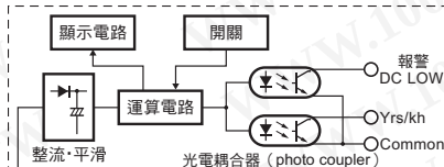
同步型 ( S8VS-09024A 型、S8VS-09024B 型 )
