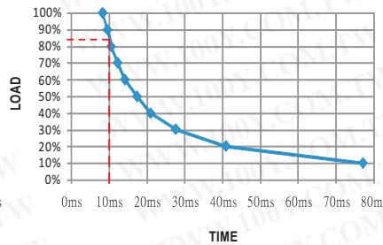
RSD-200C-24
