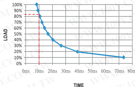
RSD-200C-24
