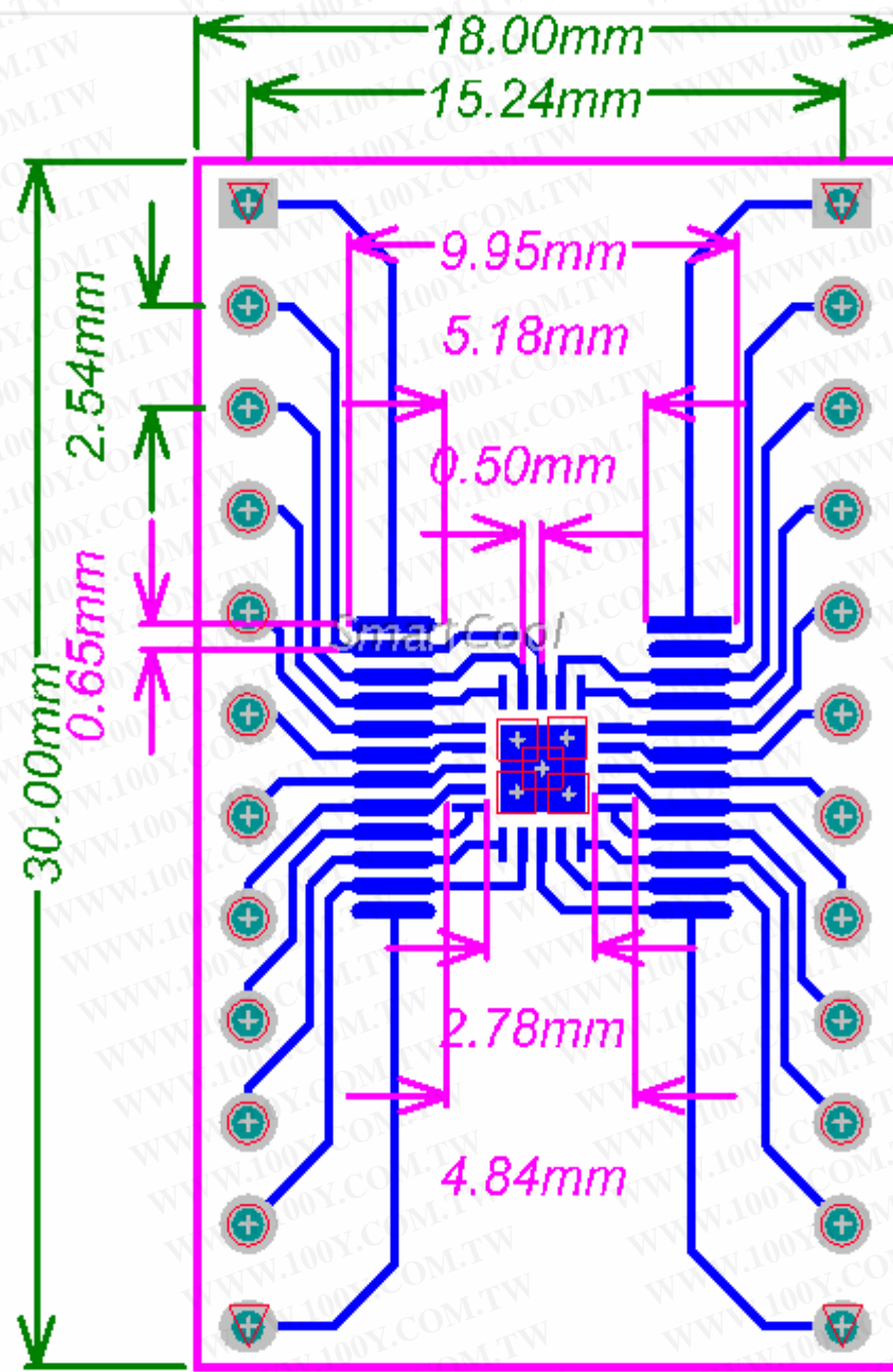
上图为<背面>：MSOP24/SSOP24/TSSOP24 & QFN20 焊盘间距 Pitch：0.65mm & 0.5mm DIP：2.54mm
