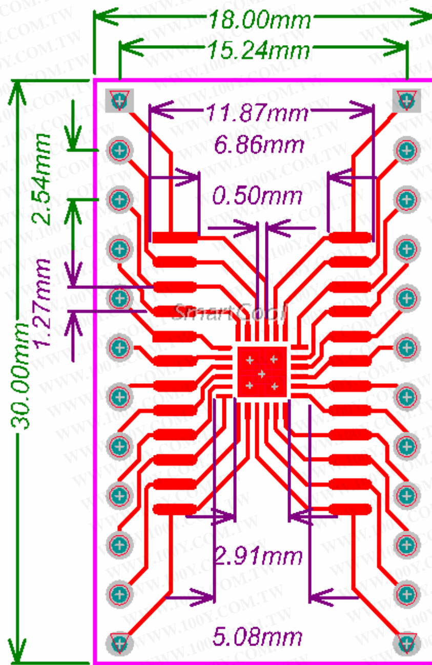
上图为<正面>：SO24/SOIC24/SOP24 & QFN24 焊盘间距 Pitch：1.27mm & 0.5mm DIP：2.54mm
