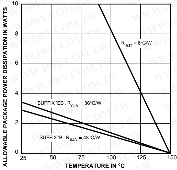
Dwg. GP-004-1A
