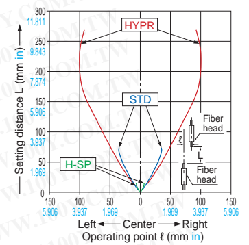
FT-E23
