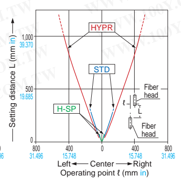
FT-H30-M1V-S
