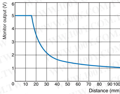
Reflective E32-DC200
