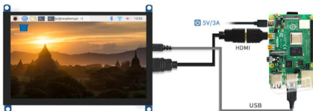
接入树莓派Raspberry Pi 4
