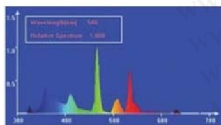
三波長燈管D-EX色光譜圖
