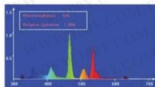
三波長燈管N-EX色光譜圖
