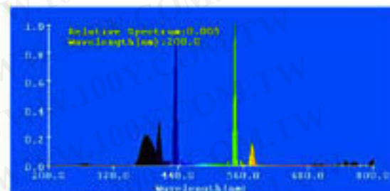
捕蟲燈管光譜圖
