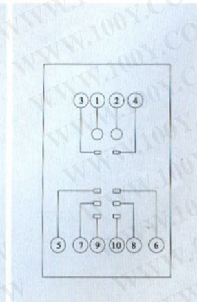
线路图 · Inter connection
