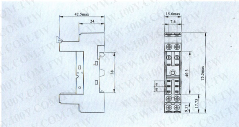
安装尺寸 · Mounting Dimension
