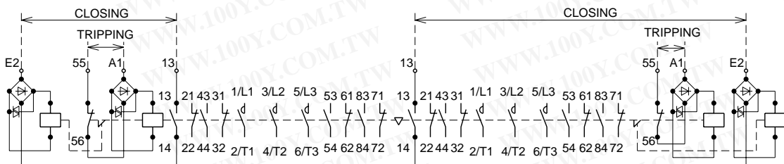
SL(D)-2xN600, N800
