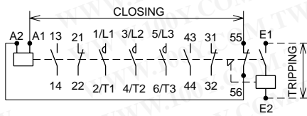
SL(D)-N21, N35
