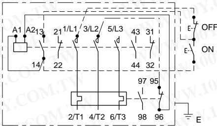
MS-N50~N150
