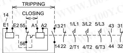
SL(D)-N80~N400
