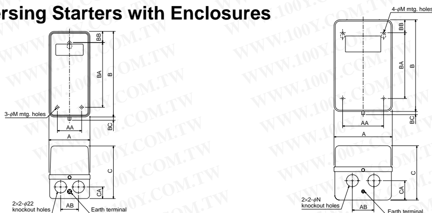
MS-N10(KP)-N21(KP)
