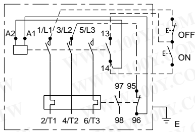
MS-N10, N11
