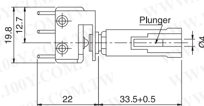
Fig. 15. Microswitch
