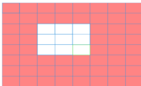
图 4.5 设置区域
