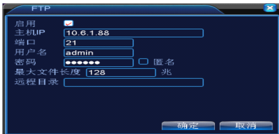
4.28 FTP 设置
