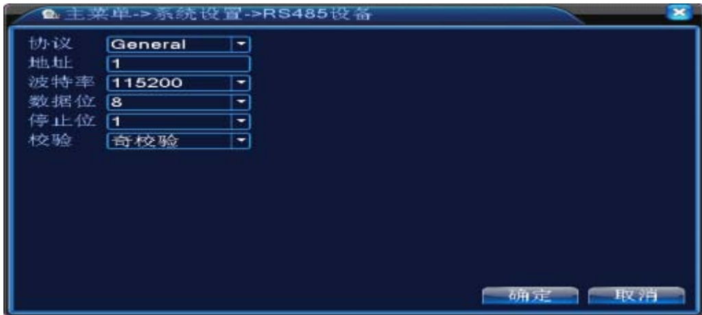
4.38 R485 设备
