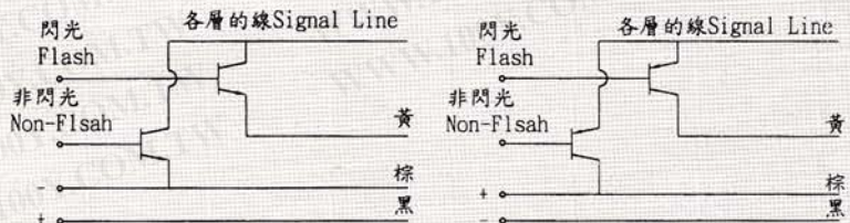
DC 12/24V NPN型配線圖
