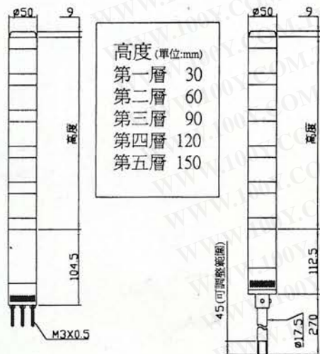
D-直付式孔位尺寸圖
