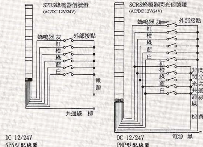
配線圖
