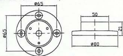
R-塑膠圓盤尺寸圖
