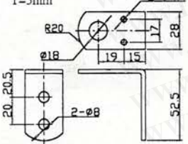
PB-鐵架式尺寸圖(可選用)
