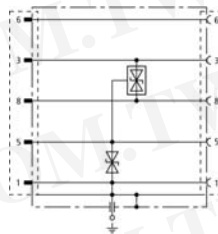
Basic circuit diagram FS 9E PB 6
