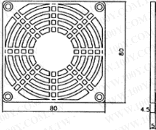
PG-80 FOR 80mm FAN
