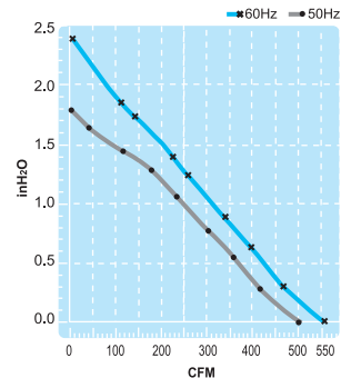
(Centrifugal Fan)
