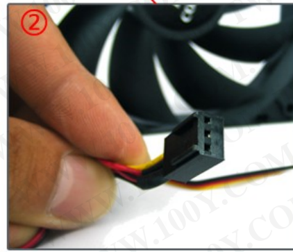
标准主板3针接口，支持测速功能
