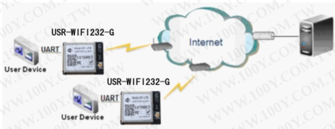
Figure 29. 远程连接应用图示
