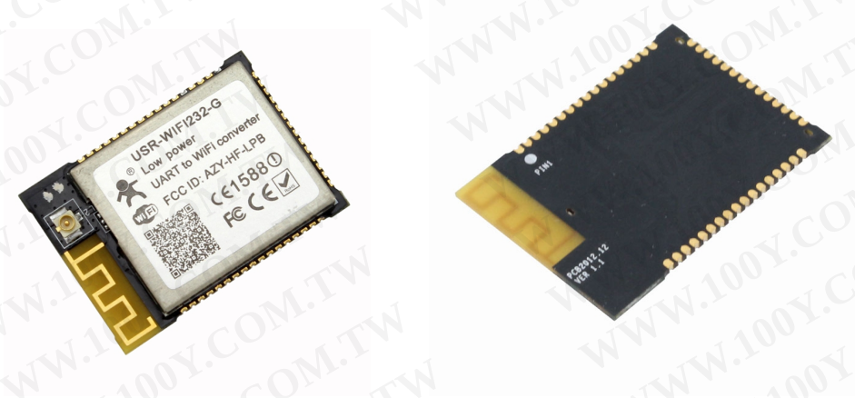
Figure 1. USR-WIFI232-G 外观图
