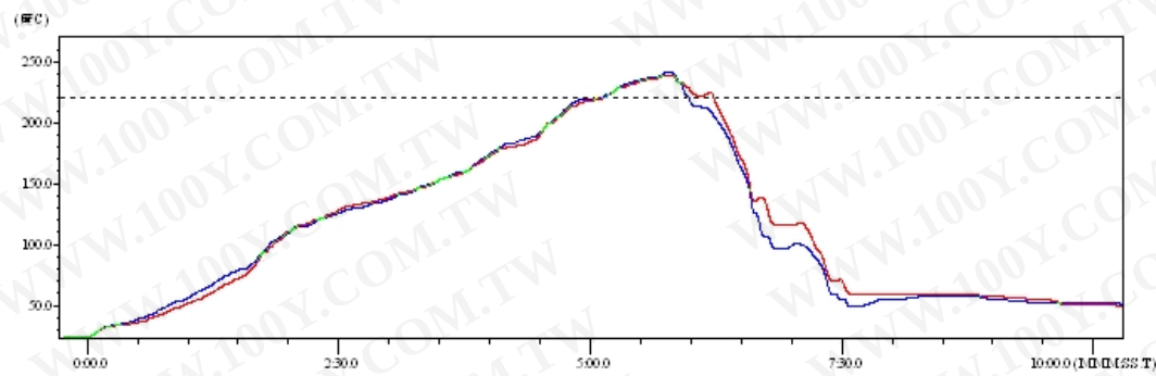
Figure 34. 回流焊焊接温度曲线图
