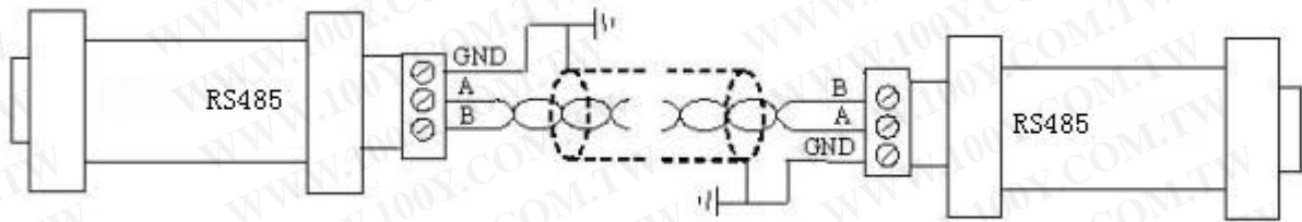
接線圖
