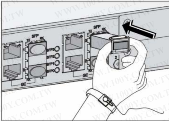
图1-4 SFP 模块安装示意图
