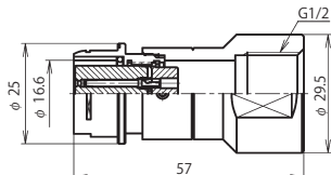
NR-20 ■ -GAdF1/2 (注)
