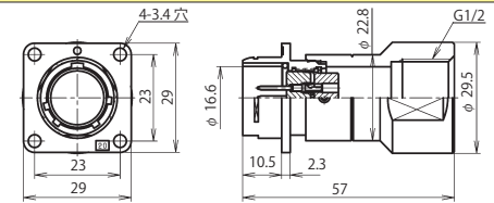
NR-20 ■ -GAd(F)M1/2 (注)
