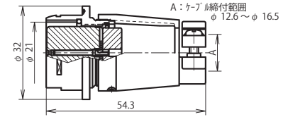
NR-24 ■ -AdF
