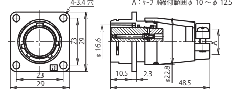
NR-20 ■ -Ad(F)F
