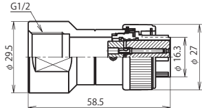
NR-20 ■ -GPF1/2 (注)
