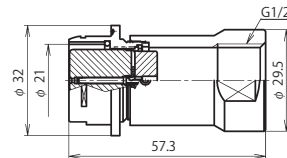
NR-24 ■ -GAdF1/2 (注)
