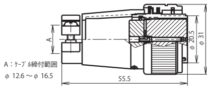
NR-24 ■ -PF
