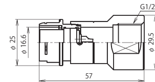
NR-20 ■ -GAdF1/2 (注)
