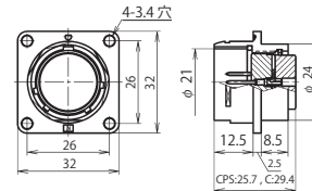
NR-24 ■ -RM
