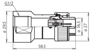
NR-20 ■ -GPM1/2 (注)
