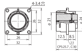
NR-24 ■ -RF
