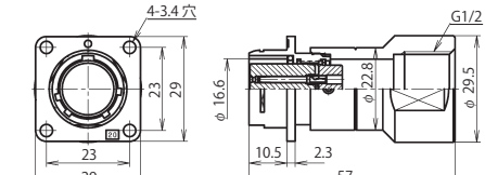
NR-20 ■ -GAd(F)F1/2 (注)
