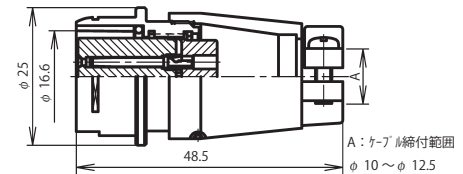
NR-20 ■ -AdF
