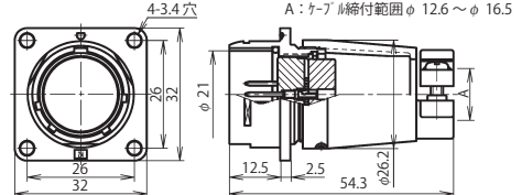
NR-24 ■ -Ad(F)M
