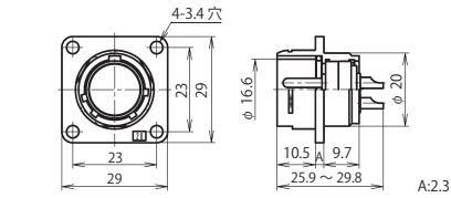
NR-20 ■ -RM
