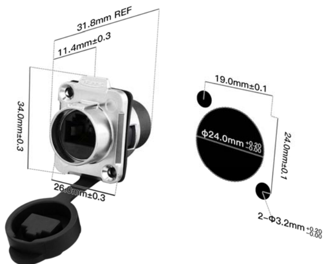
两孔法兰插座
