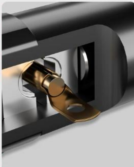
2. 端子裝入壓接模中間
