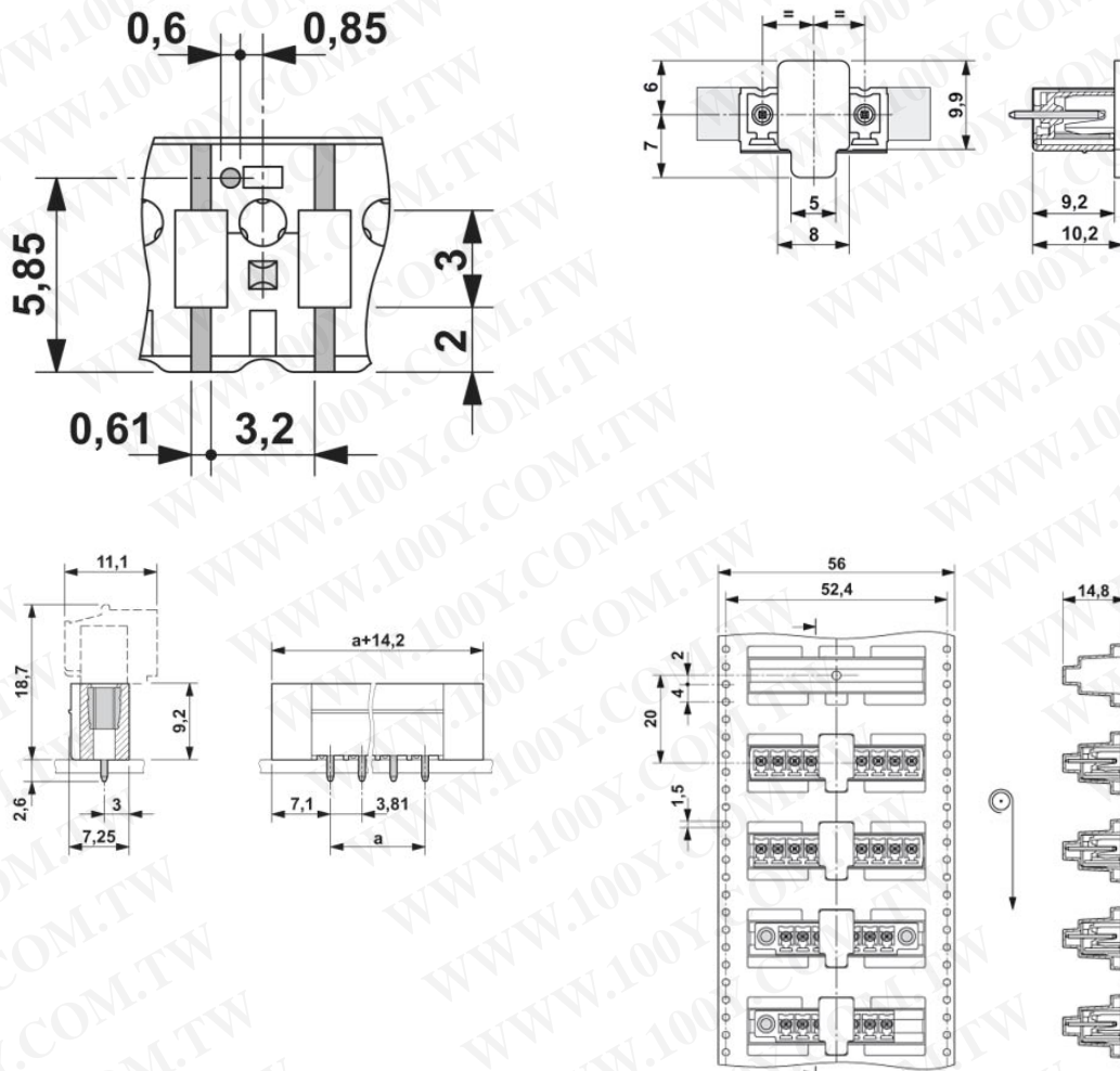
尺寸图
