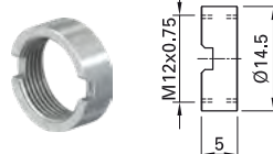
MUR/M12x0,75
