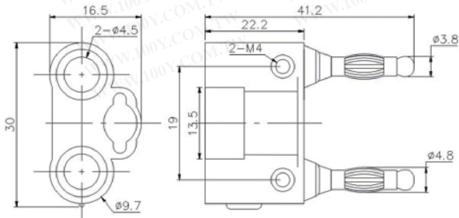
外形尺寸图:
