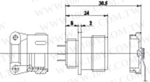
X30型插座
