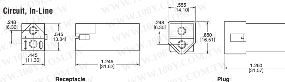
Receptacle
