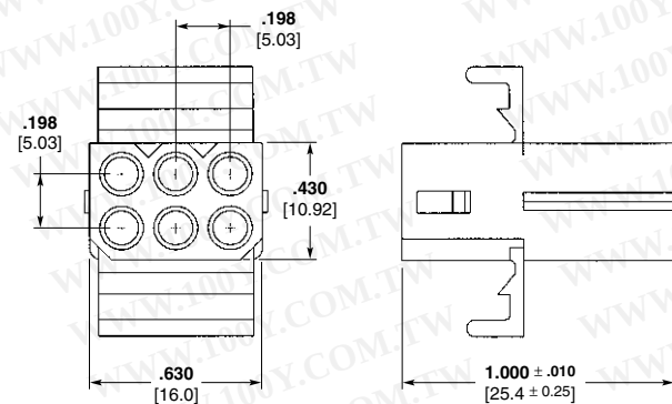
Receptacle
