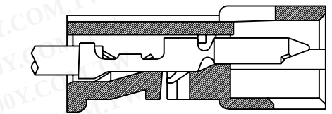
断面 E-E SECT. E-E
