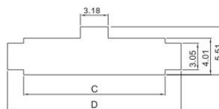
插座 RECEPTACLE HOUSING (43640)
