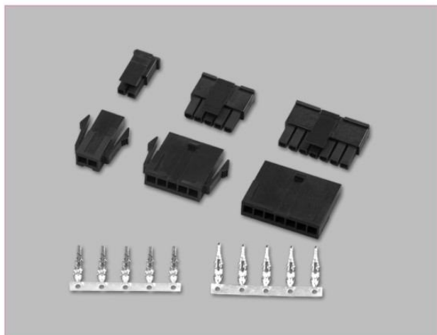
端子 TERMINAL (43030、43031)
