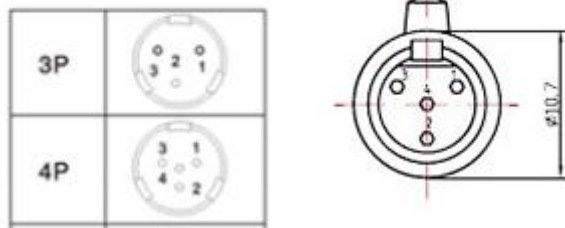
接觸件位置排列
