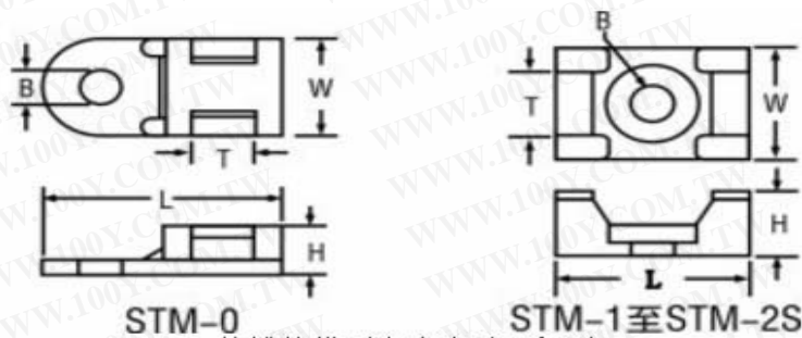
扎线扎带固定座产品工程图
