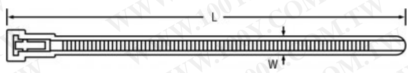
活用式尼龍束線帶 RCT 系列工程圖
